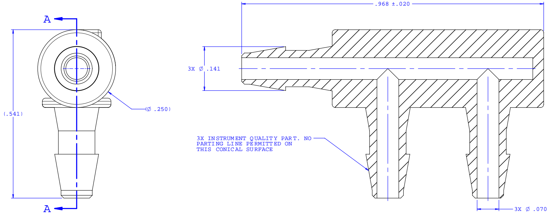
SECTION A-A
