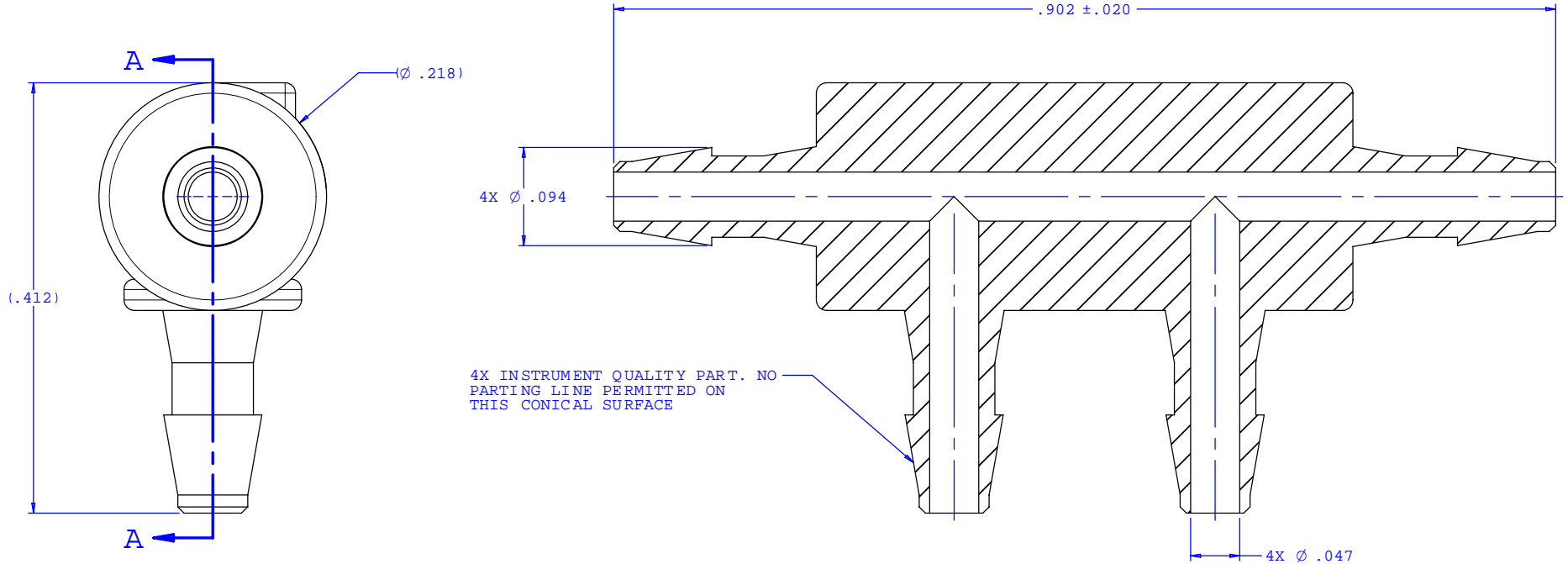
SECTION A-A
