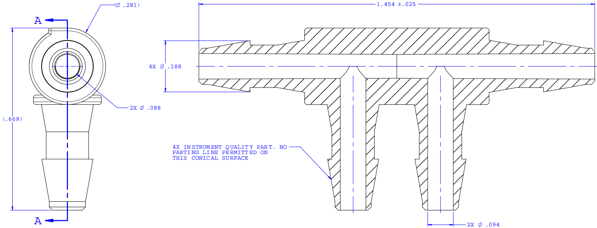
SECTION A-A
