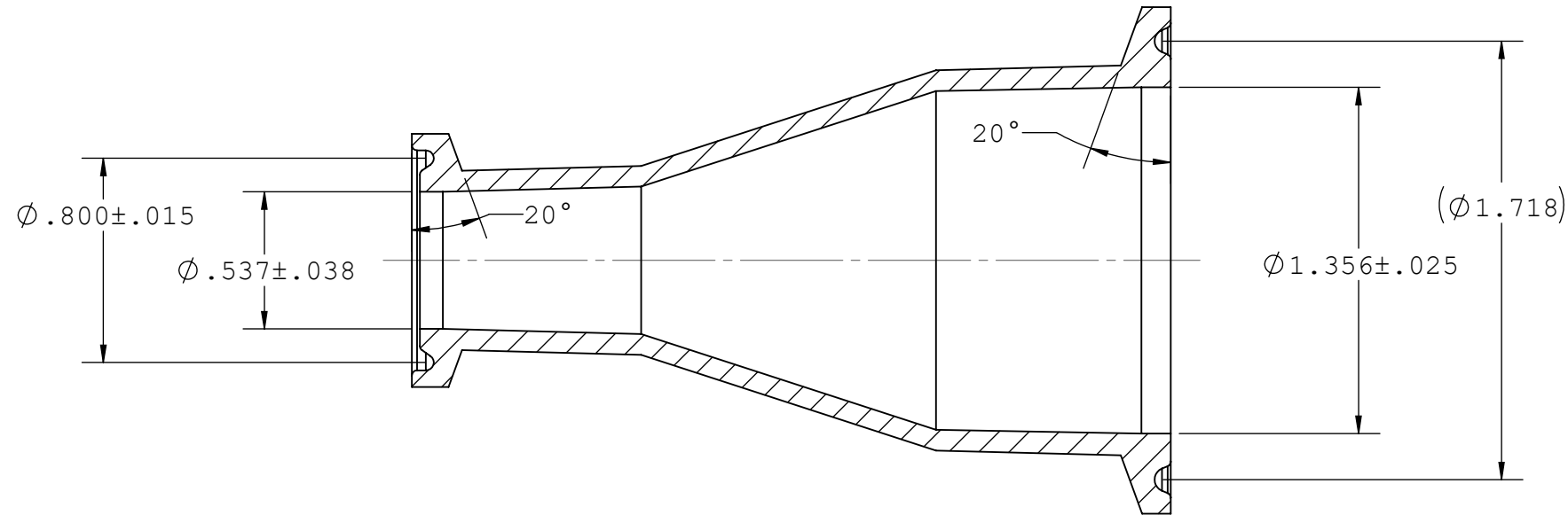
SECTION A-A
