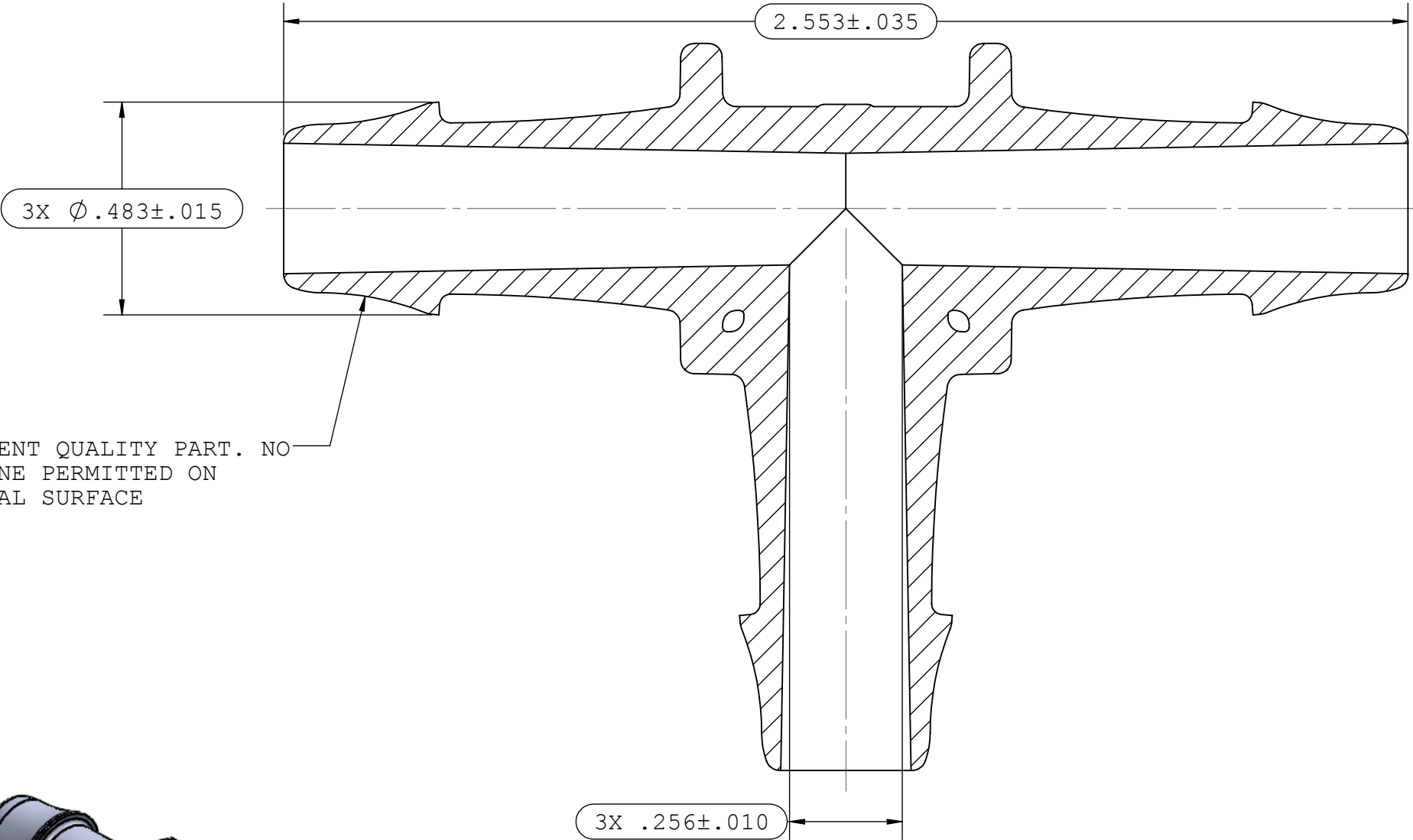
SECTION A-A
