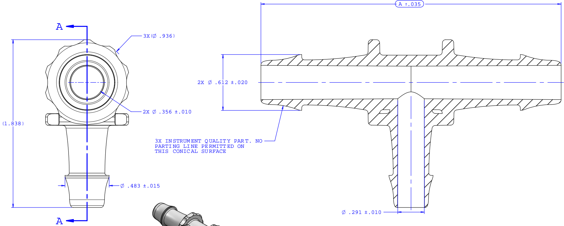
SECTION A-A
