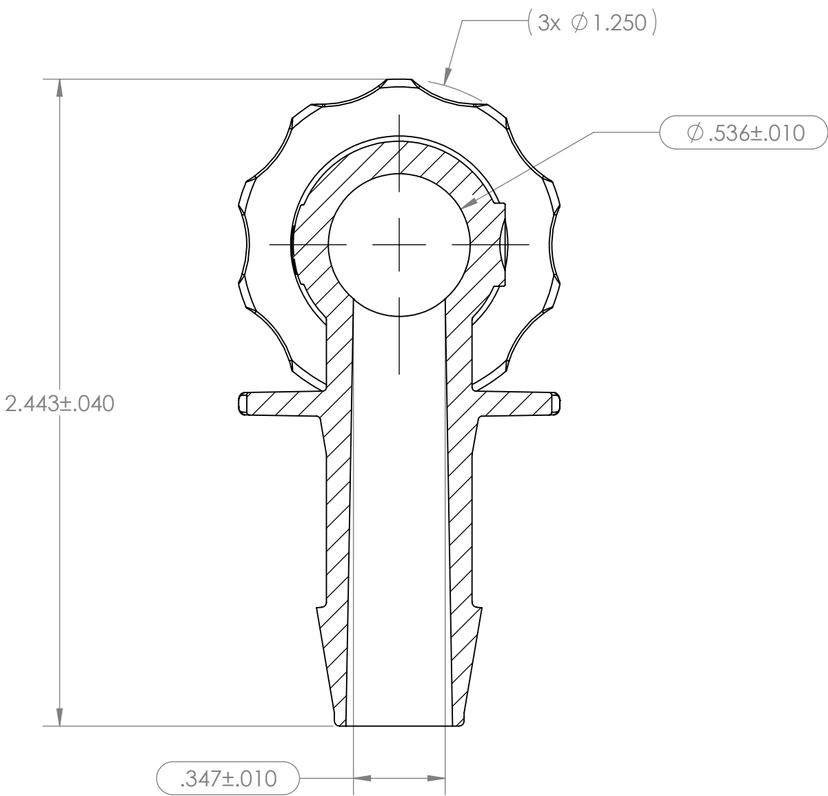
SECTION A-A
