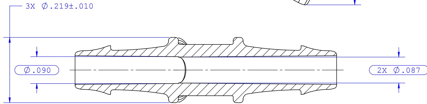
SECTION A-A
